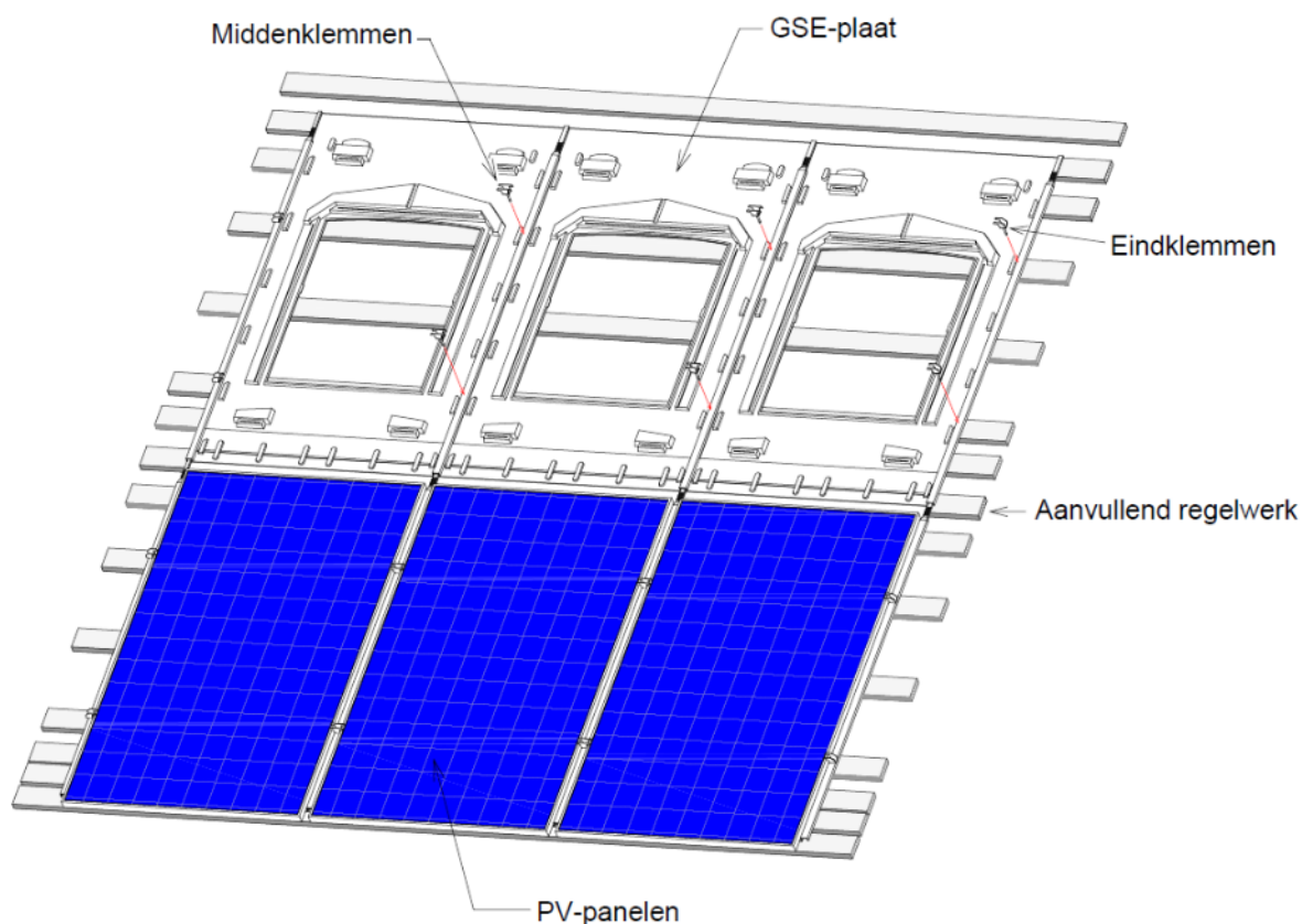
Figuur 1 – Systeemopbouw (exploded-view)
