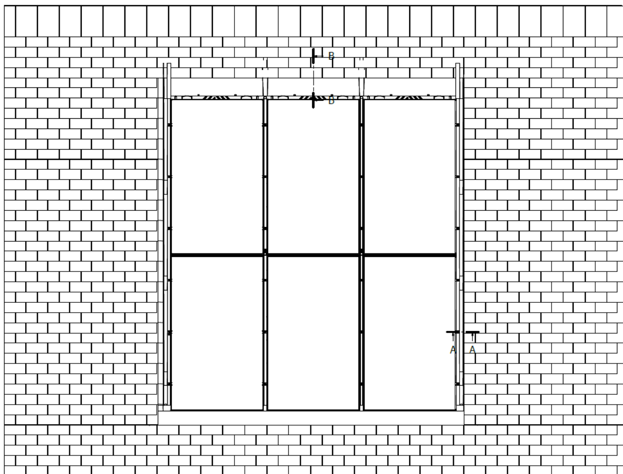
Figure 33 – Mise en place des éléments de couverture (kit A-2)
