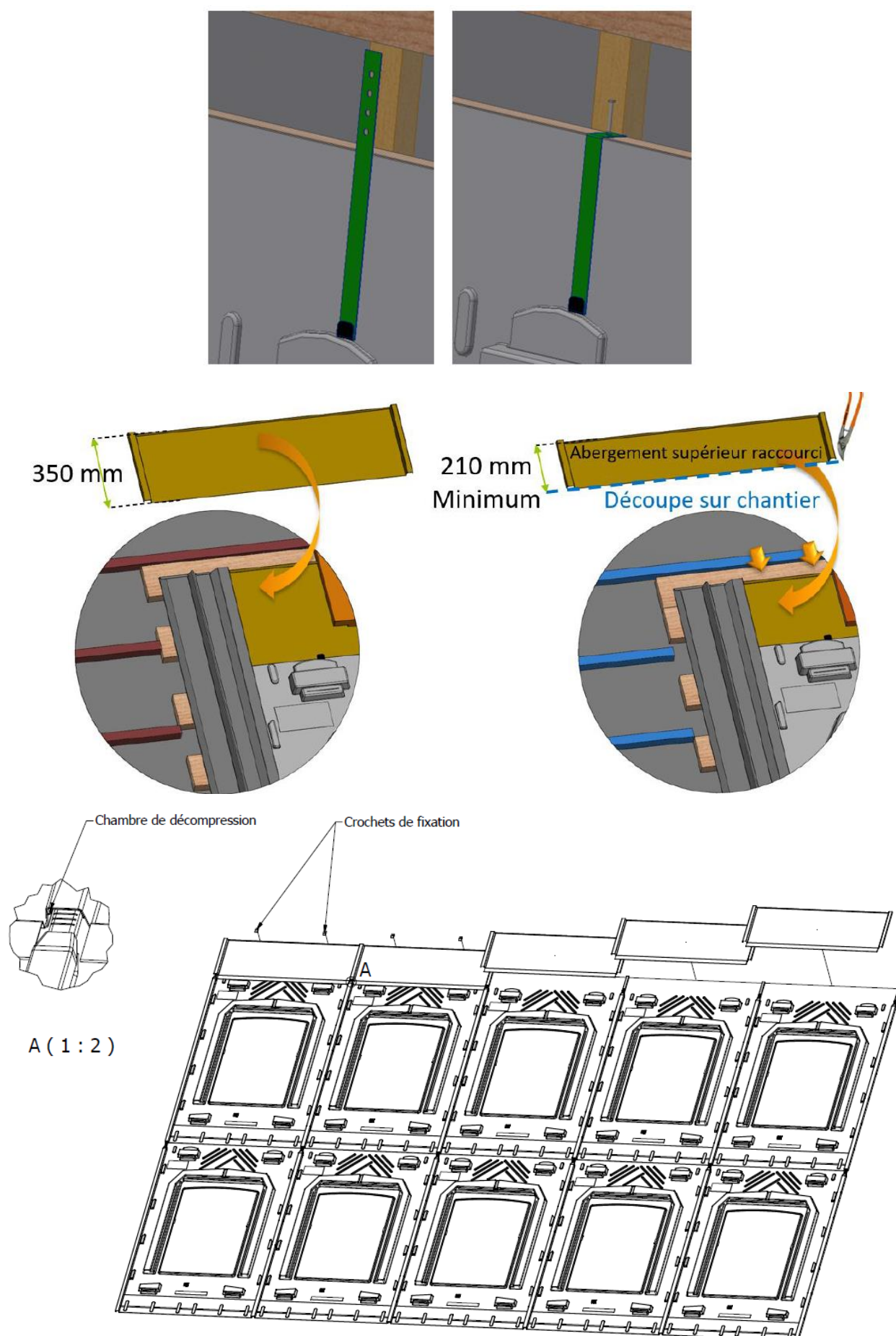
Figure 24 – Pose des abergements supérieurs (kit TS-2)
