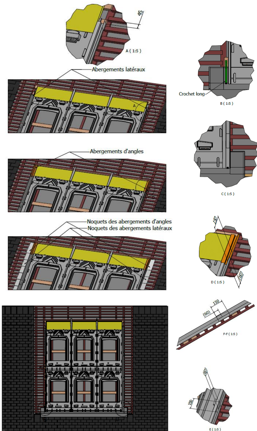
Figure 32 – Pose des abergements latéraux et d'angles supérieurs (kit A-2)
