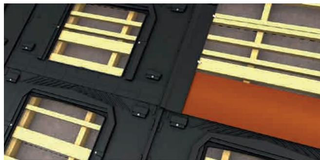
Anbringen der seitlichen Verblechung
