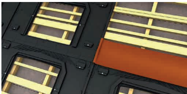
Aufbringen des formbaren Zinkbandes
