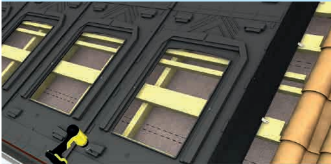
Vorbohren der Wannen: 4 Befestigungspunkte
