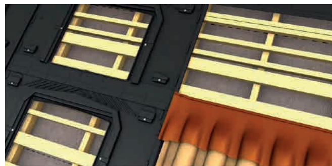
Anbringen des flexiblen Zinkbandes
